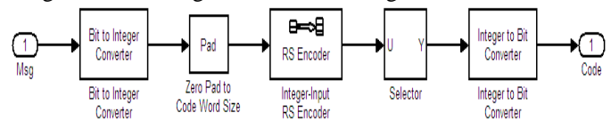
Fig: 4 Block Encoder
