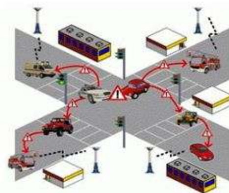
Fig.1 VANET Scenario
