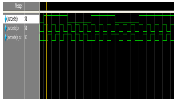
Manchester Coding
