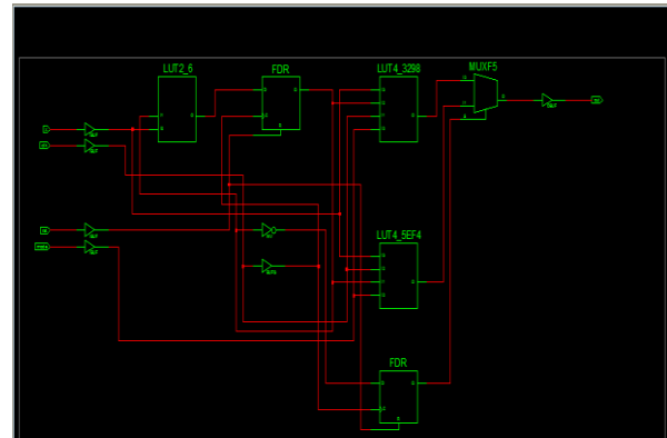
Manchester Coding
