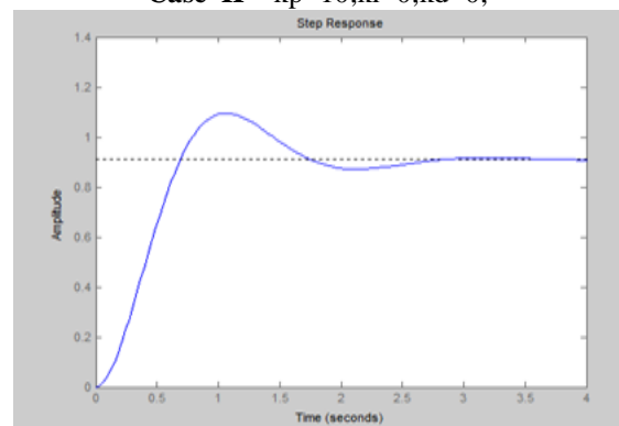
Case II k_p=10;k_i=0;k_d=0;
