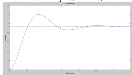
Case II k_p=10;k_i=0;k_d=0;
